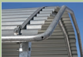
Sveobuhvatna zaštita krovnog ruba
